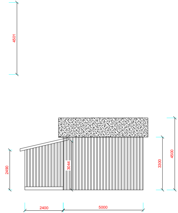
VÄSTERFASAD
