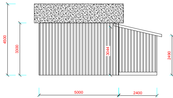
ÖSTERFASAD
